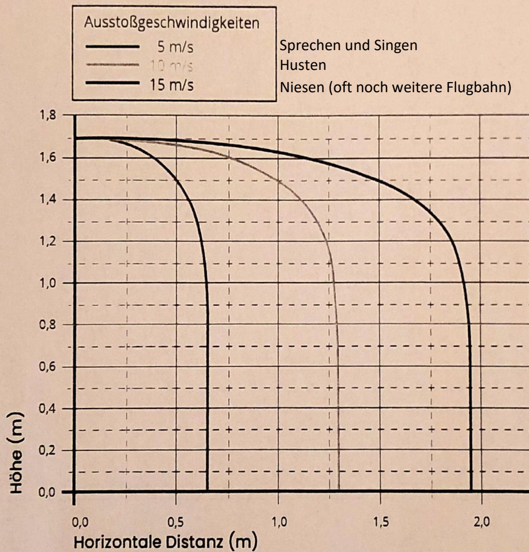
Abbildung 3: Flugbahnen von Tröpfchen eines Durchmessers von 200 \mu\text{m} und der Dichte von Wasser, die in einer Höhe von 1,70 m mit unterschiedlichen Geschwindigkeiten ausgestoßen werden (in Anlehnung an [57])
